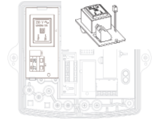
Mains module
